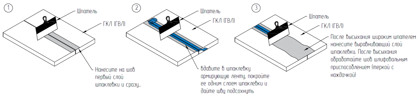
Рис. 31. Порядок шпаклевки швов между листов ГКЛ (ГВЛ) с использованием армирующей сетки
