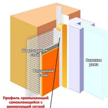
Рис.21. Профиль примыкающий с армирующей сеткой
